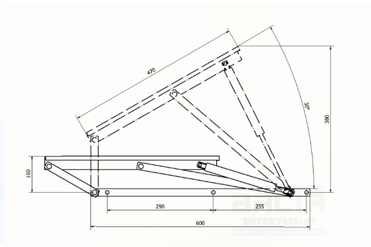
Gázrugós francia vasalat (párban)
