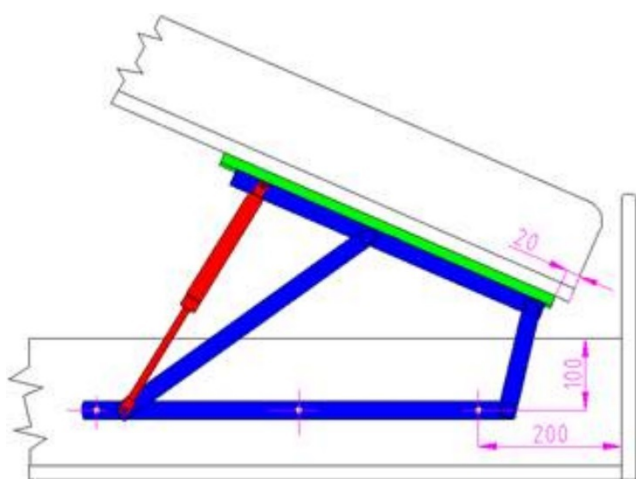
Gázrugós francia vasalat (párban)
