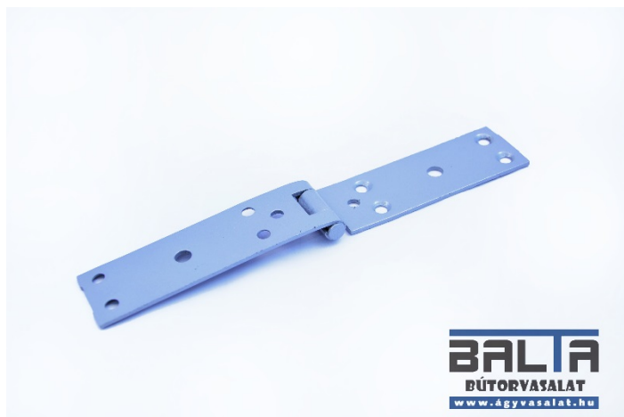
Fordított összerakású ládazsanér
