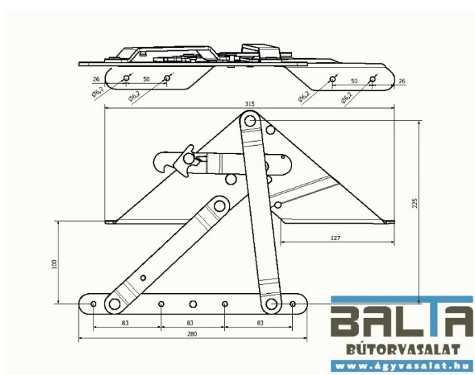
Alacsony kattanós vasalat (párban)
