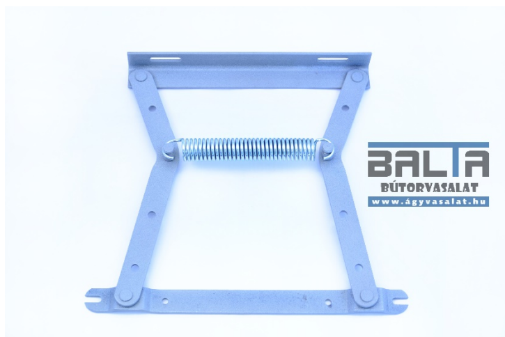
Alacsony íves kiemelő vasalat rugóval (párban)
