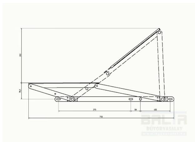
Slicelt pamlagemelő vasalat sínrel, rugóval (párban)
