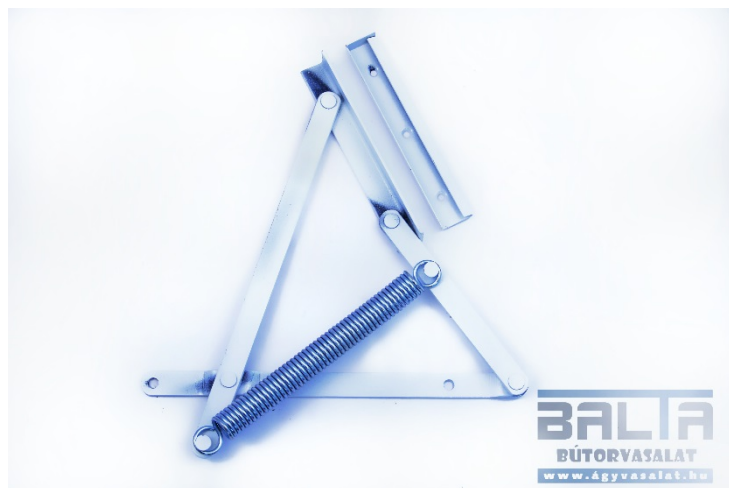
Kétszemélyes átlapolt vasalat, rugóval (párban)
