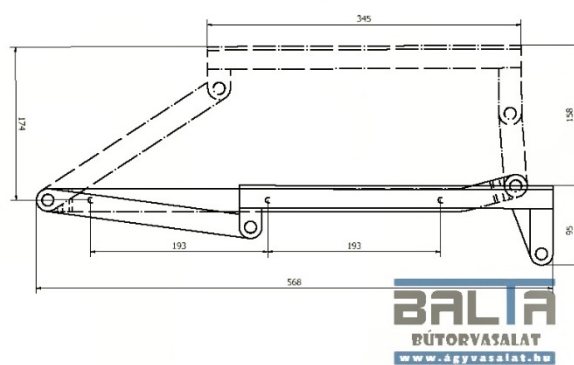
Gabi vasalat (párban)
