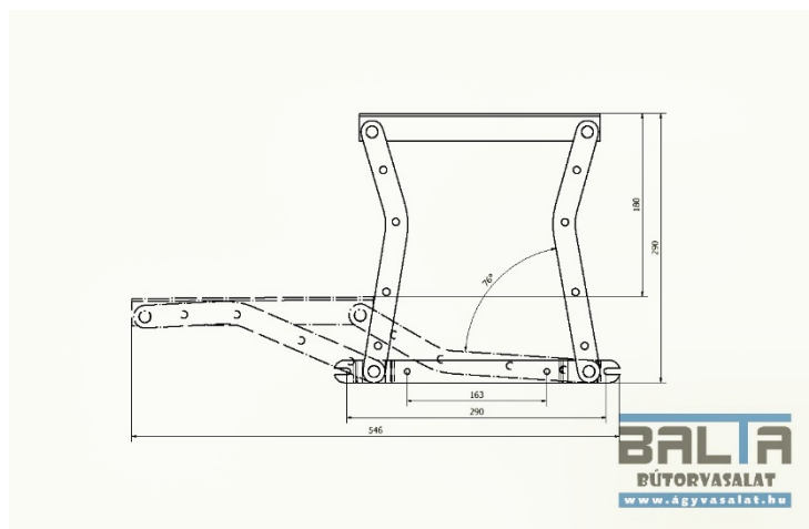
Alacsony íves kiemelő vasalat rugóval (párban)
