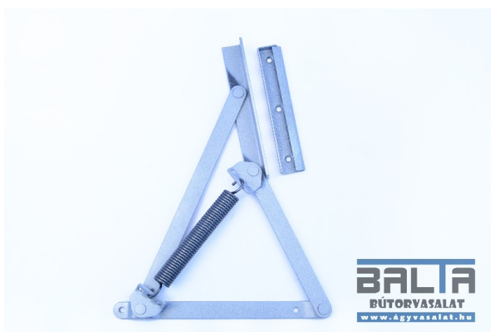
Heverő vasalat sínnel, rugóval (párban)
