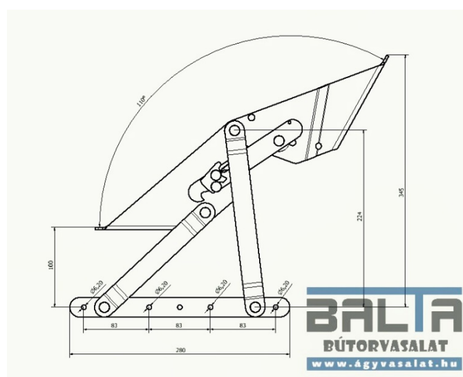
Alacsony kattanós vasalat (párban)
