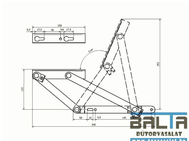
Kanapé vasalat rugóval (párban)
