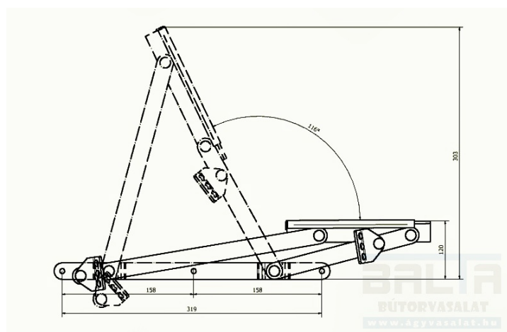
Inox vasalat sínnel, rugóval (párban)
