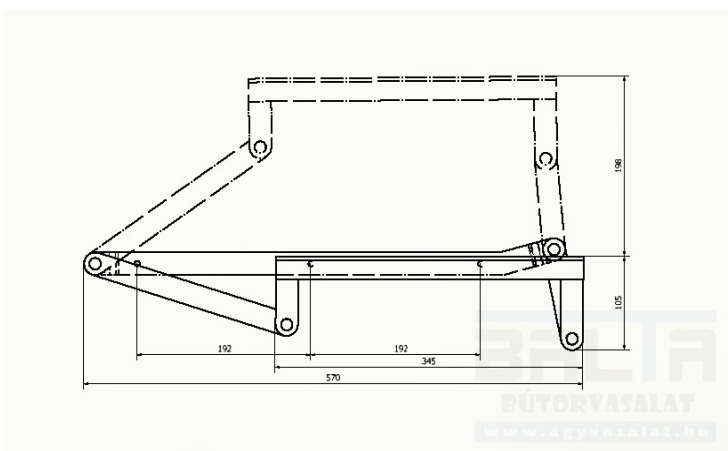
Gabi vasalat (párban)
