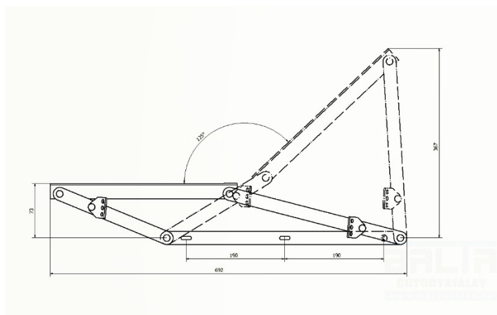
Módosított pamlagemelő vasalat, rugóval (párban)
