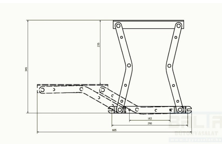
Magas íves kiemelő vasalat rugóval (párban)
