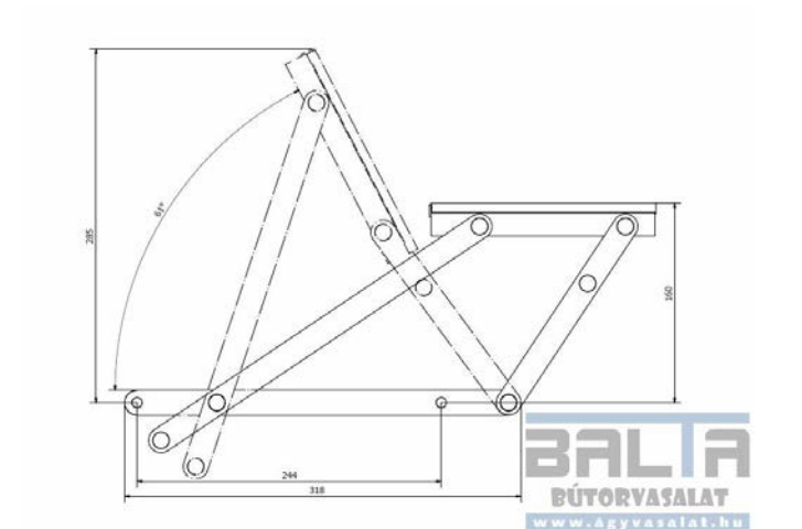
Kétszemélyes vasalat sínnel, rugóval (párban)
